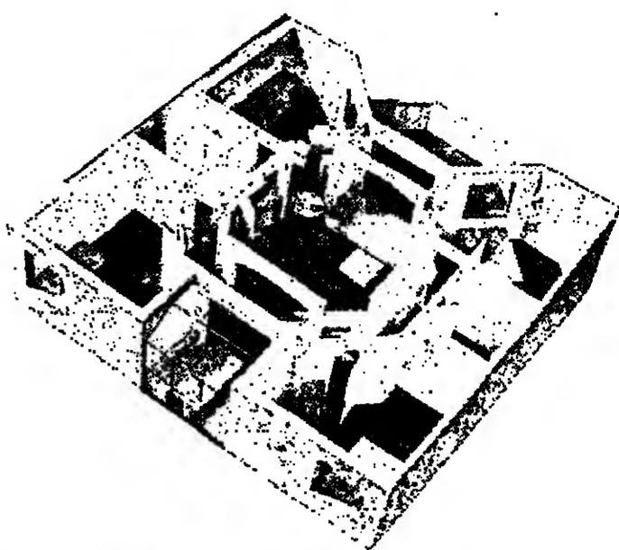
Dans le modèle « Arcade », conçu par les architectes Jean-Pierre Buffi, Yves Tiesler et Bernard Wauthier, la pièce commune est un centre, entouré d'arades que l'on peut éventuellement cloisonner. Elle est éclairée, côté rue, par une vérande et, côté jardin, par une terrasse-patio. La cuisine et les chambres sont situées aux quatre coins de l'appartement. La surface de l'ensemble est de 80 mètres carrés environ, à quoi s'ajoutent la terrasse et la vérande.
